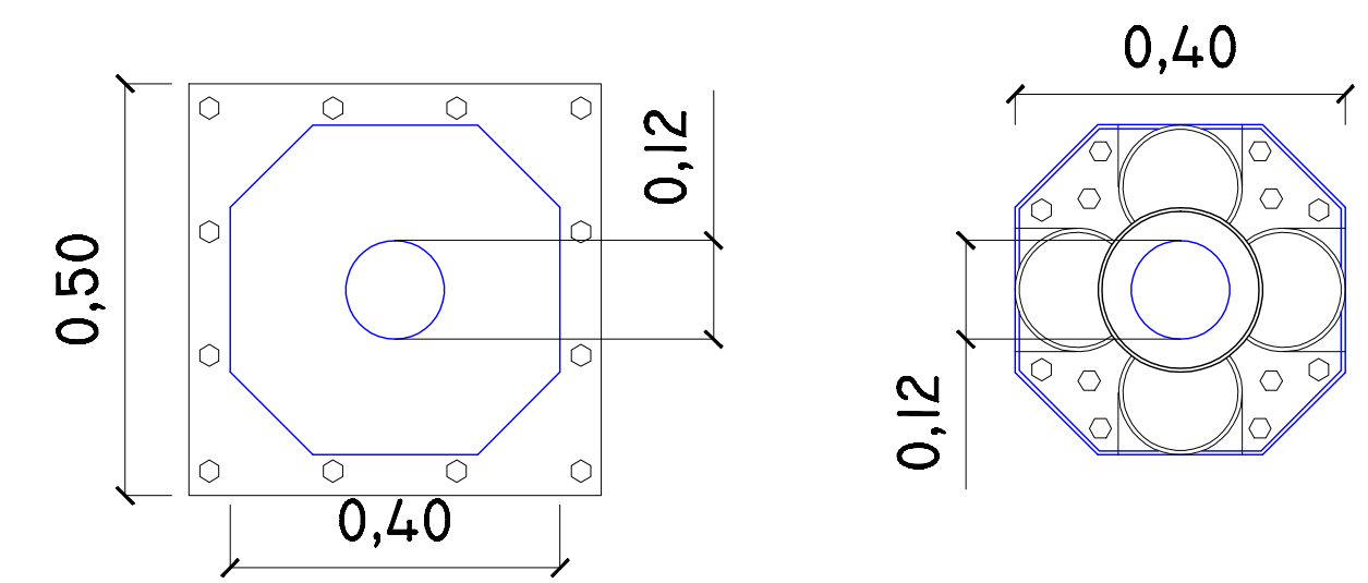
DETALHE 01 BASE DO PILAR ESCALA 1 : 10
